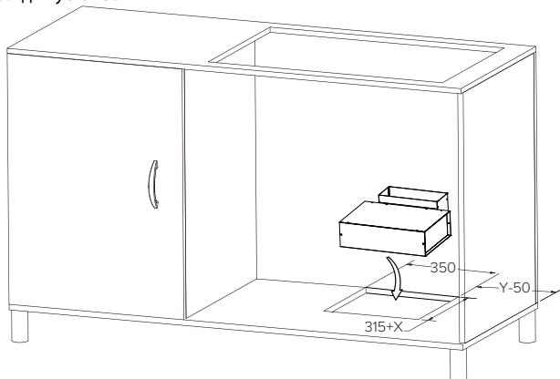
Рис.5 Размеры выреза вентиляционной системы
